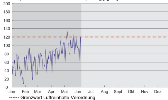
Ozon, maximale Stundenmittelwerte pro Tag [ \mu\text{g}/\text{m}^3 ]
