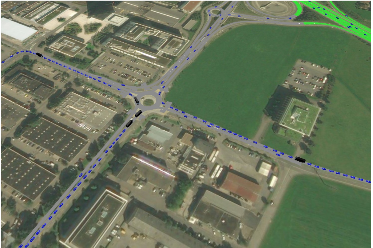
Abbildung 25 Staubildung gemäss Vissim beim Kreisell «Forren», Referenzzustand 2030 ASP
