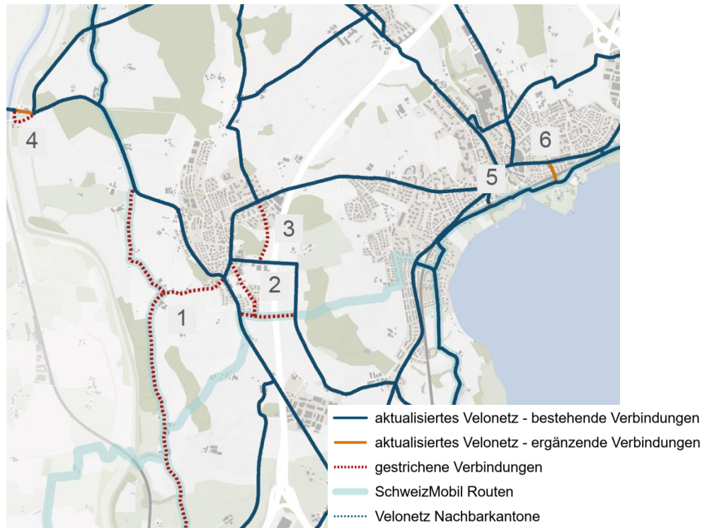
Abbildung 27: gestrichene und ergänzte Verbindungen Rotkreuz/Hünenberg
