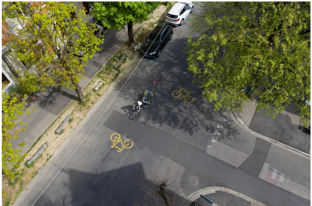
Abbildung 35: Prinzip Velostrasse mit vortrittsberechtigter Führung in Tempo-30-Quartierstrassen (Aufhebung Rechtsvortritt)
