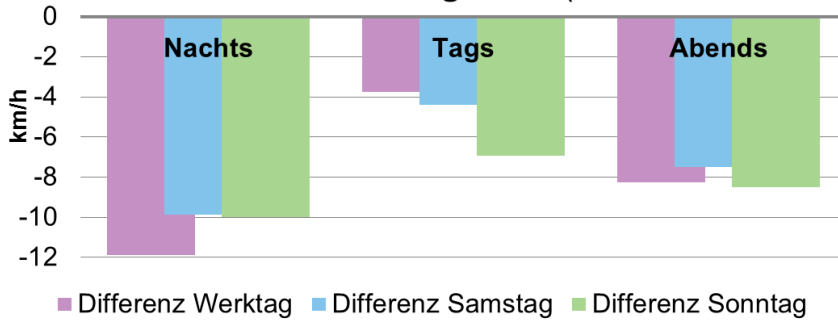
V85 Richtung Kolin (Messstelle Casino)
