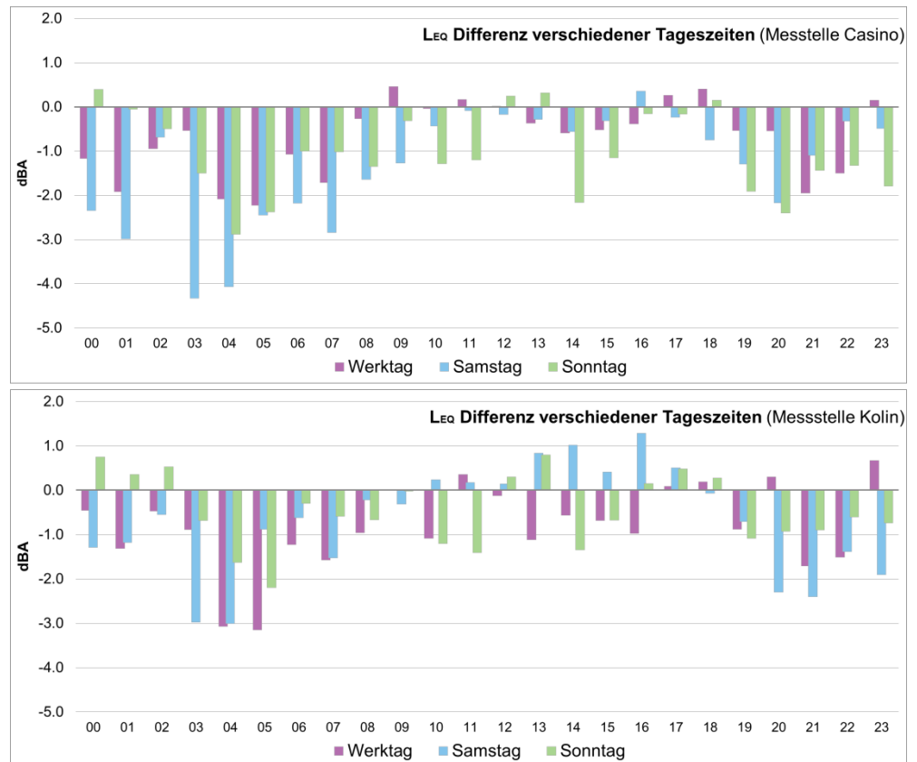
Reduktion der mittleren Lärmpegel an beiden Messstellen zu den verschiedenen Tageszeiten
