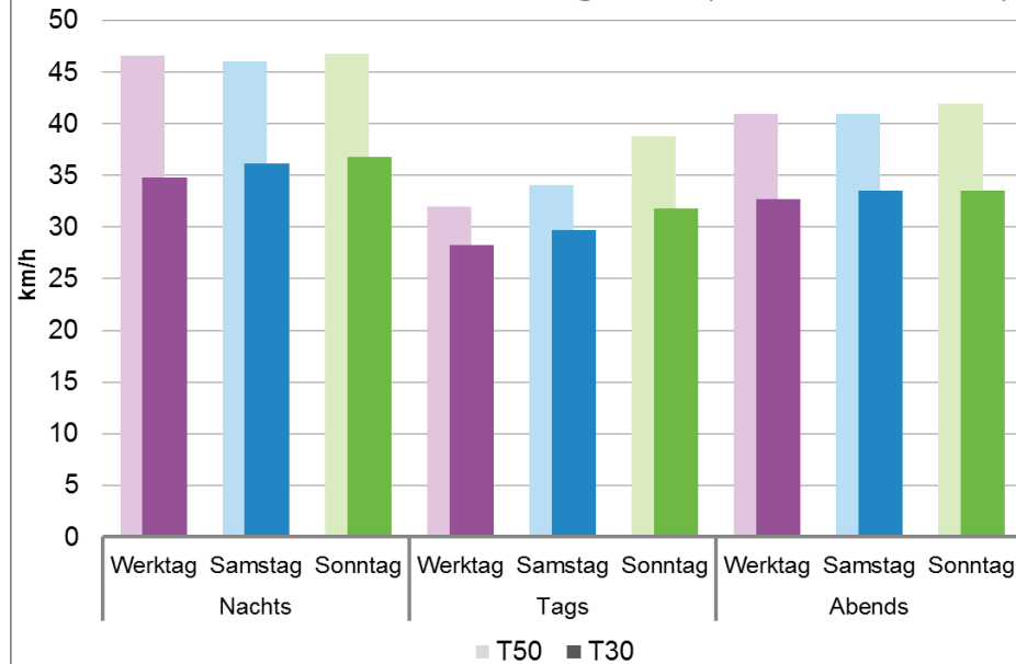
v85 Richtung Kolin (Messstelle Casino)
