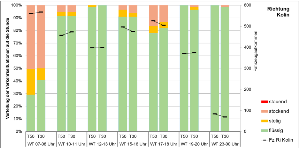
Verteilung der Verkehrsflusssituationen auf ausgewählte Stunden Werktags
