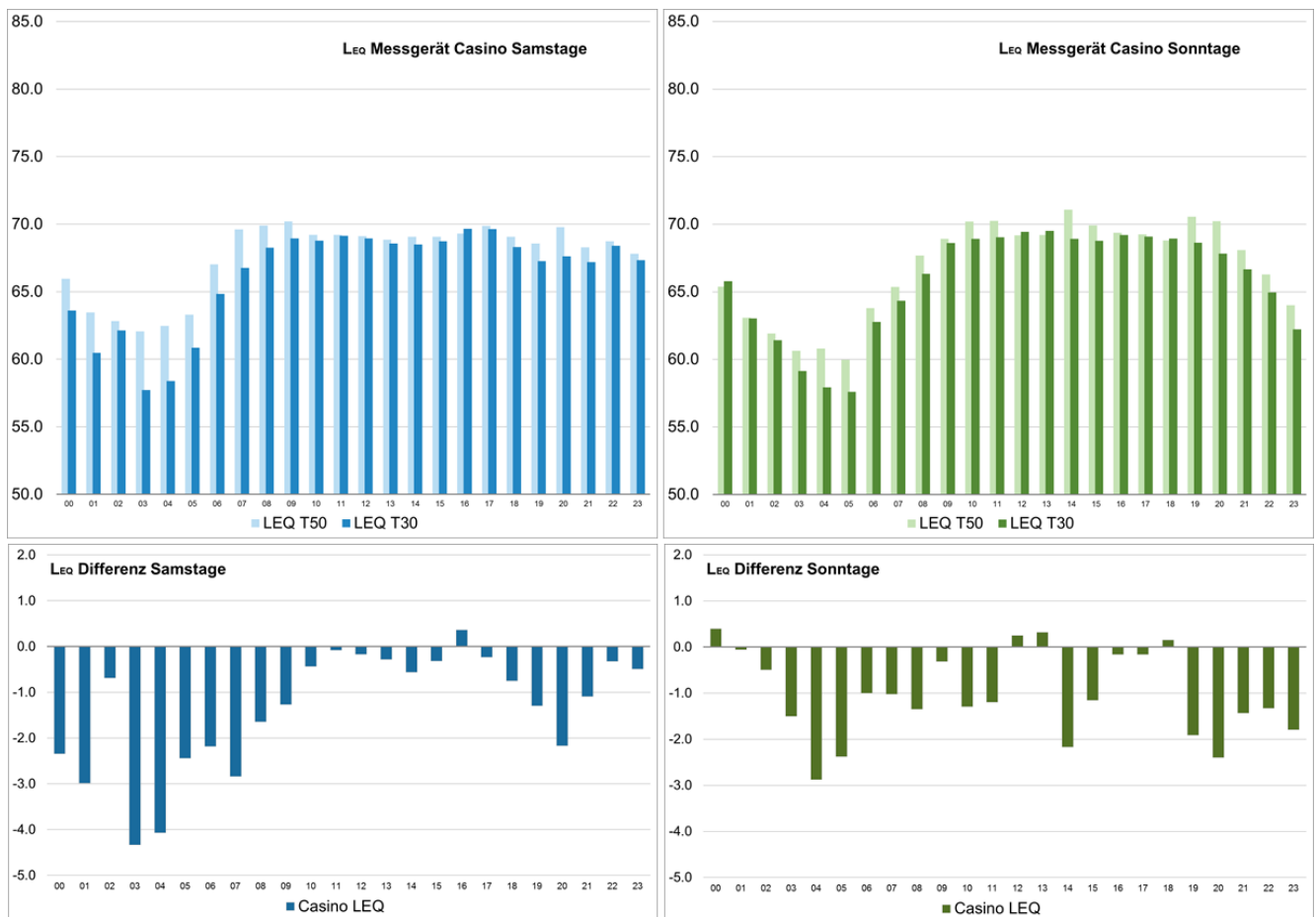
Gemittelter Pegel am Wochenende
