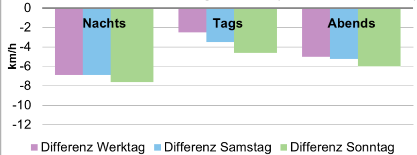
V85 Richtung Casino (Messstelle Casino)
