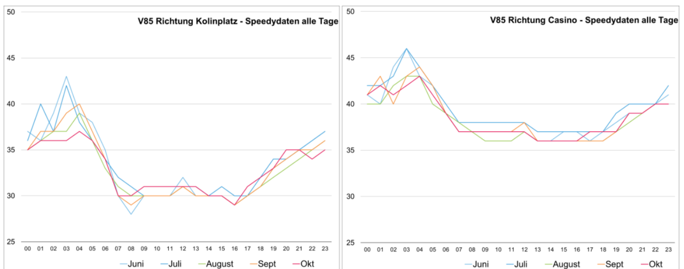
Monatliche Speedy-Daten der Geschwindigkeiten
