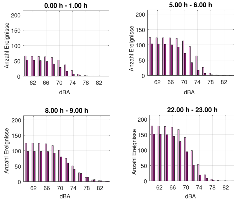
Anzahl von Ereignissen hoher Lärmpegel in ausgewählten Stunden (Summenkurve der Ereignisse pro Werktag)
