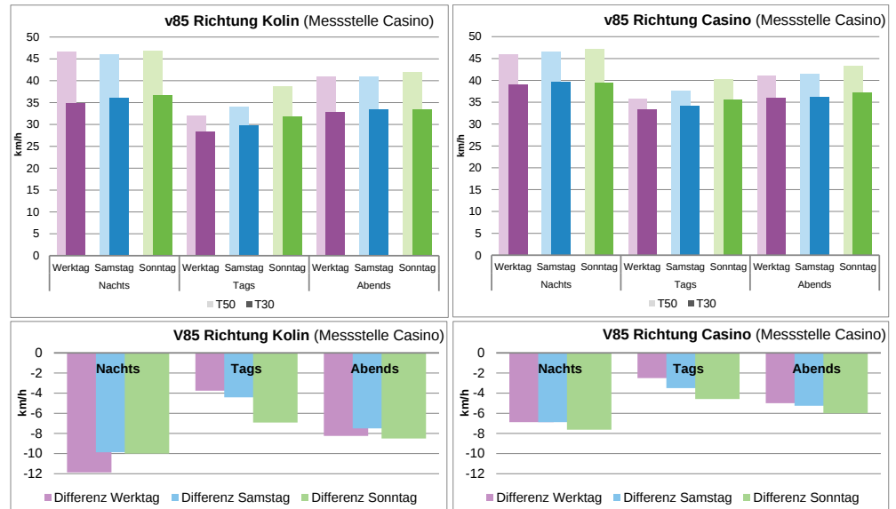
V85 verschiedener Tageszeiten und ihre Veränderung mit T30
