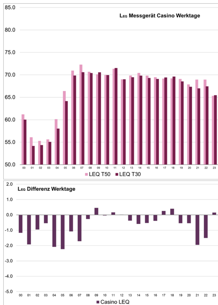
Gemittelter Pegel Werktags
