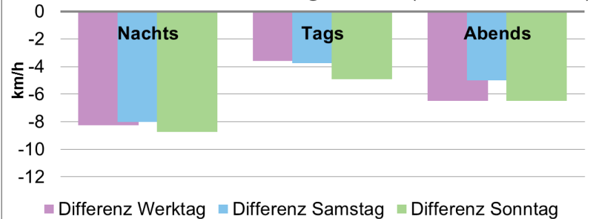
V85 Richtung Casino (Messstelle Kolin)
