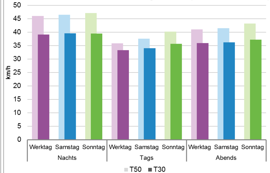
v85 Richtung Casino (Messstelle Casino)
