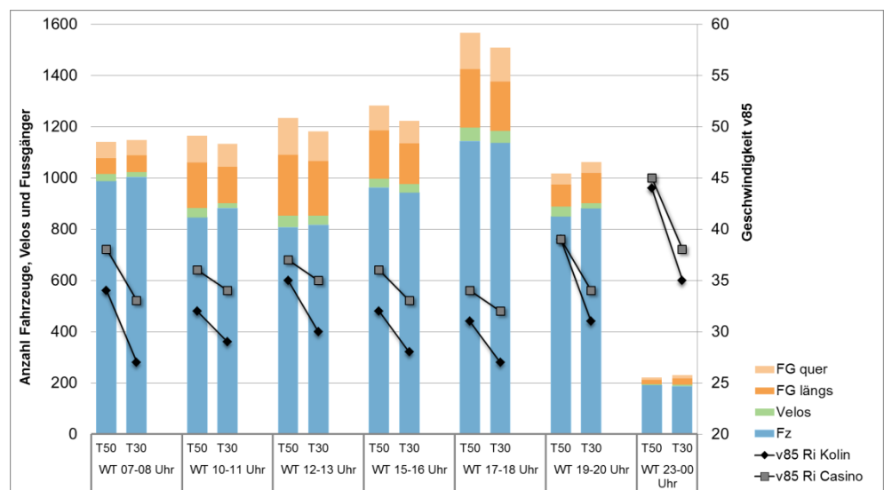
Anzahl Fahrzeuge, Velos und Fussgänger sowie v85 in ausgewählten Stunden Werktags
