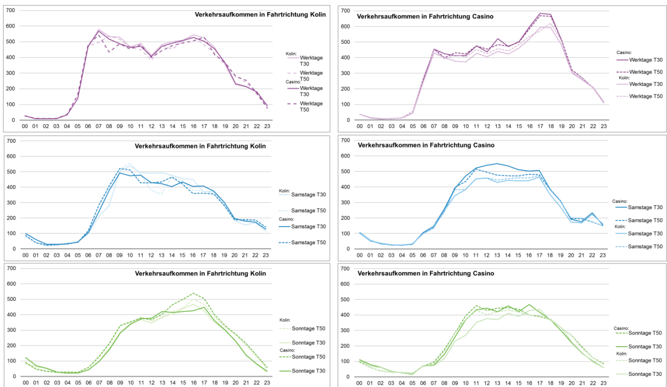
Verkehrsaufkommen in beiden Richtungen und an beiden Zählstellen
