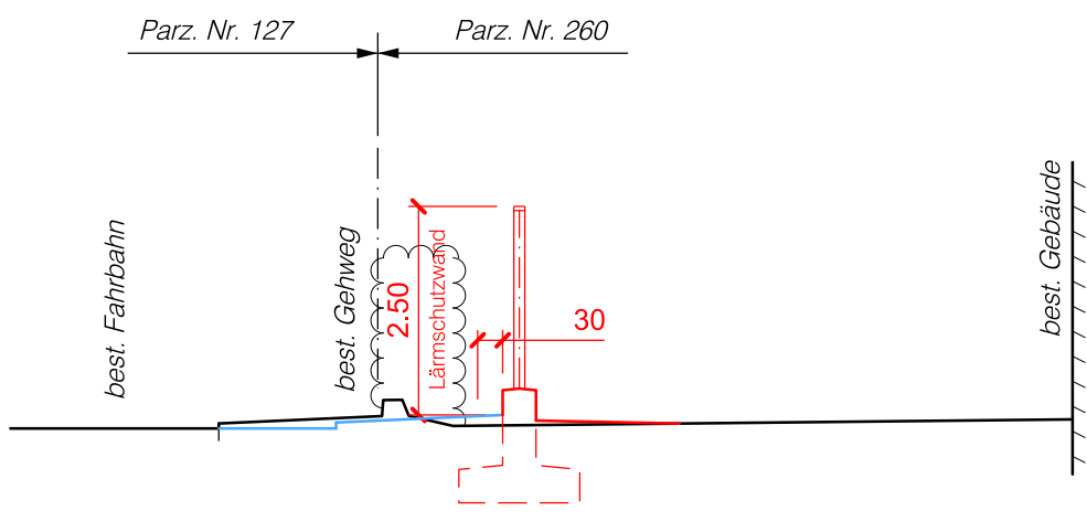
Querschnitt C - C 1:100
