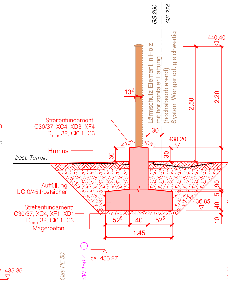
Querprofil 4 - 4 1 : 50
