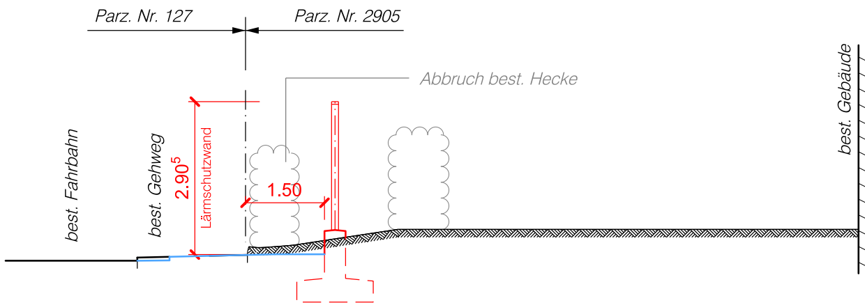
Querschnitt D - D 1:100
