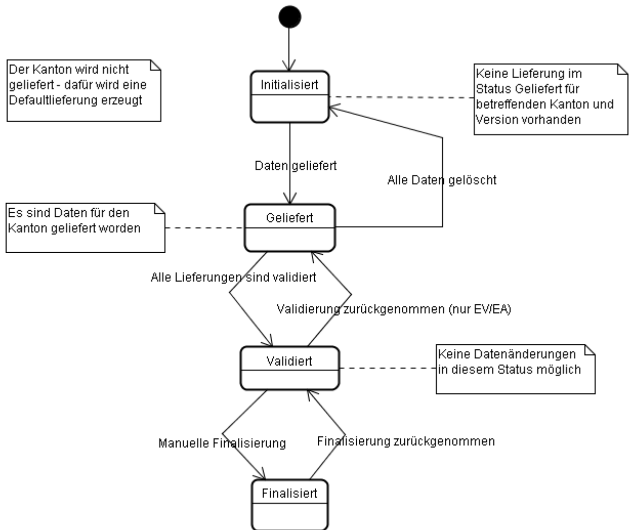
Abbildung 27: Zustandsdiagramm Kanton
