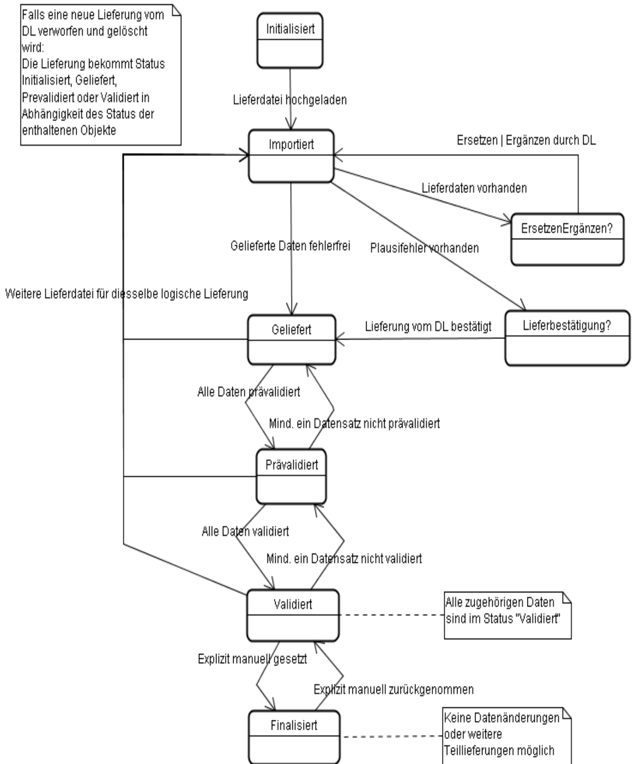
Abbildung 28: Statusübergänge Lieferung
