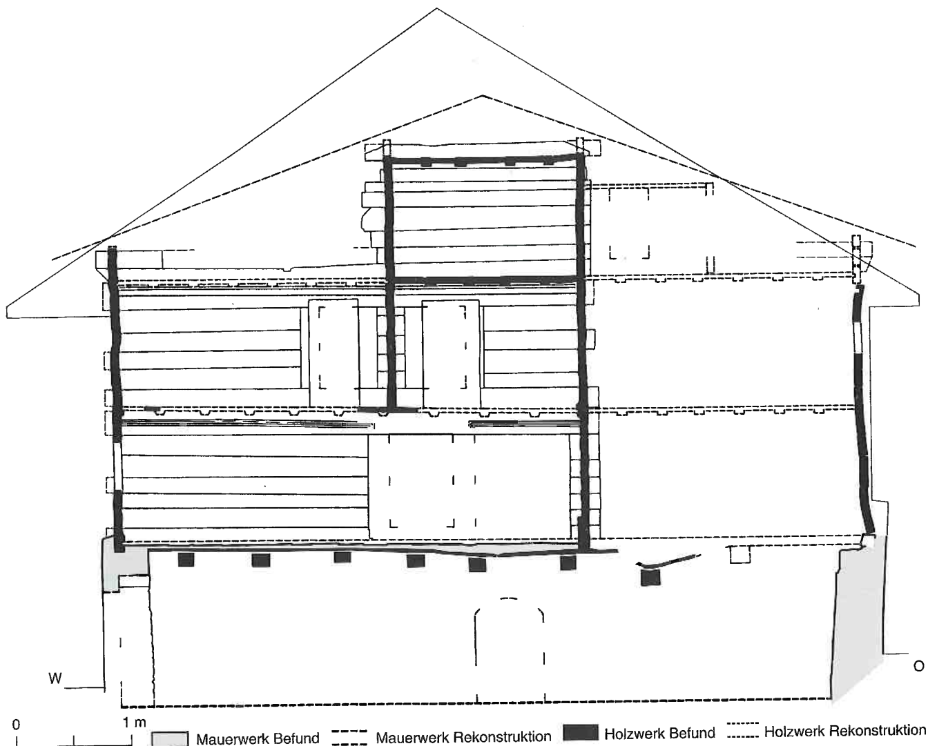
Abb. 5 Neuheim, Hinterburg, Haus «Spittel». West-Ost-Schnitt im Bereich der Erdgeschoss-Binnenmauer (Umzeichnung Hanspeter Hertli, Stand April 1991). Aufgrund des Westwandabschlusses sowie der Höhe der Firstkammer lässt sich die ursprüngliche Dachneigung rekonstruieren.
