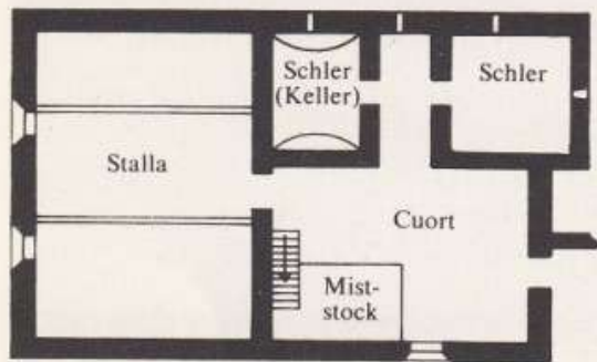
Plan suot – Untergeschoss
